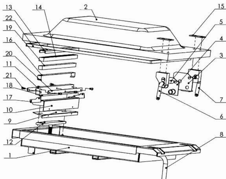
Рисунок 7.1 - Покомпонентное представление модуля вакуумной камеры
